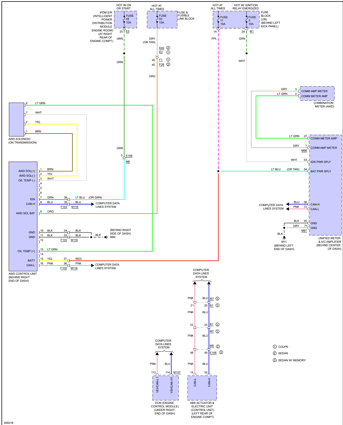
Fig 2: AWD Circuit
