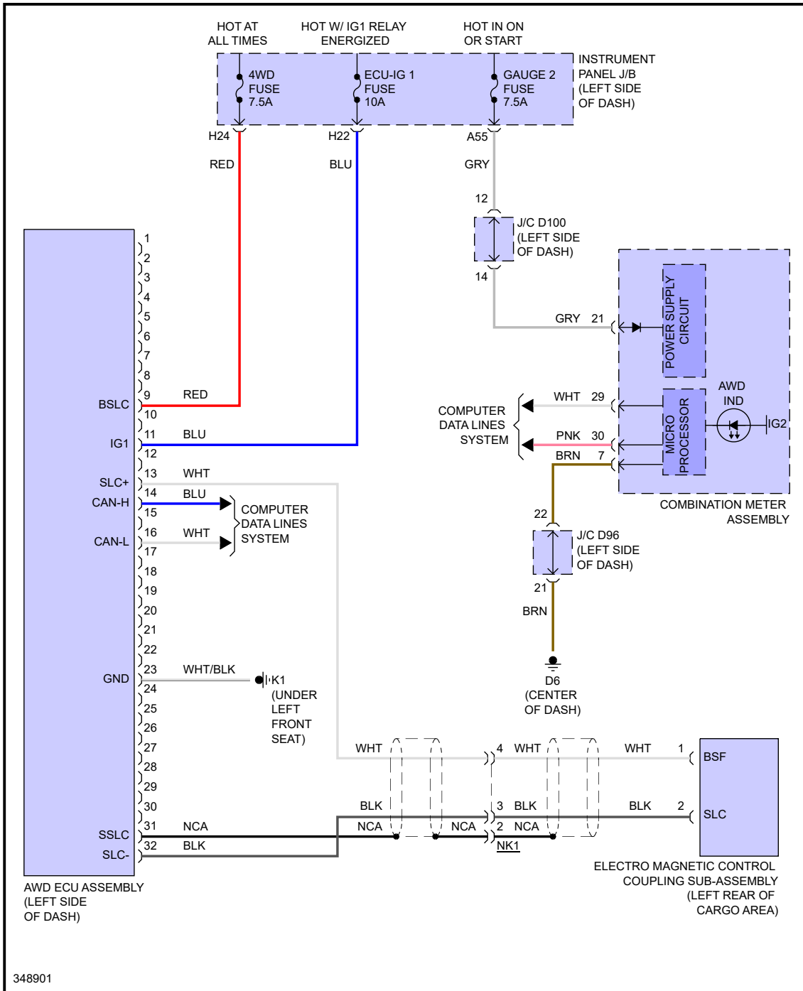
Fig 3: 2.7L, AWD Circuit
